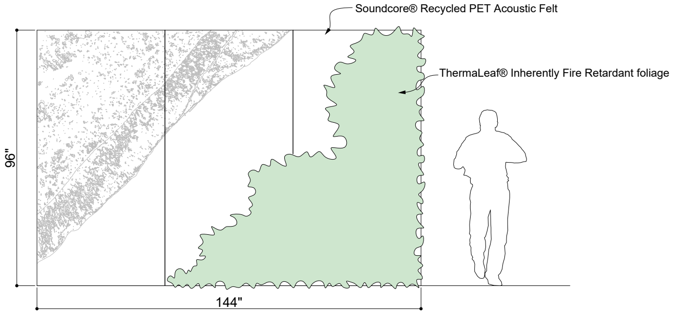
① ELEVATION 1
