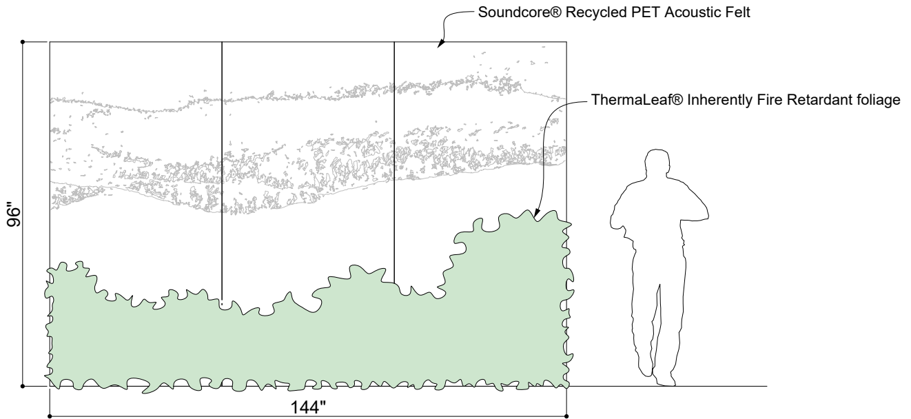
② ELEVATION 2
